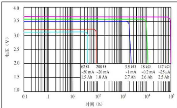
25°C放电特性曲线
