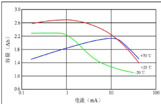
容量与电流关系曲线
