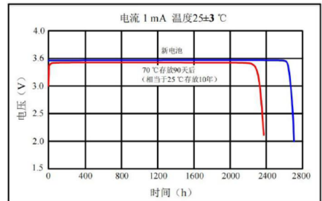
储存特性曲线
