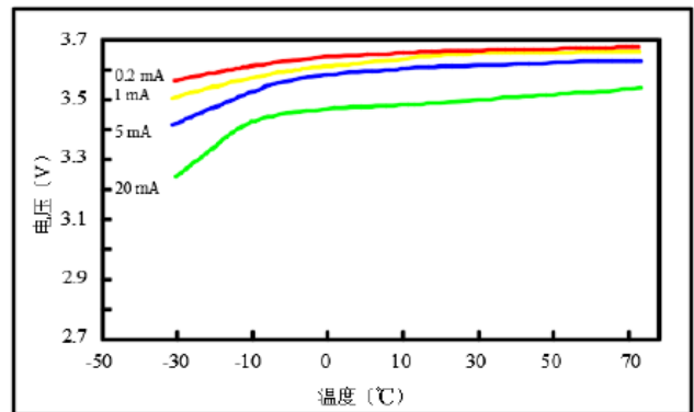
电压电流关系曲线
